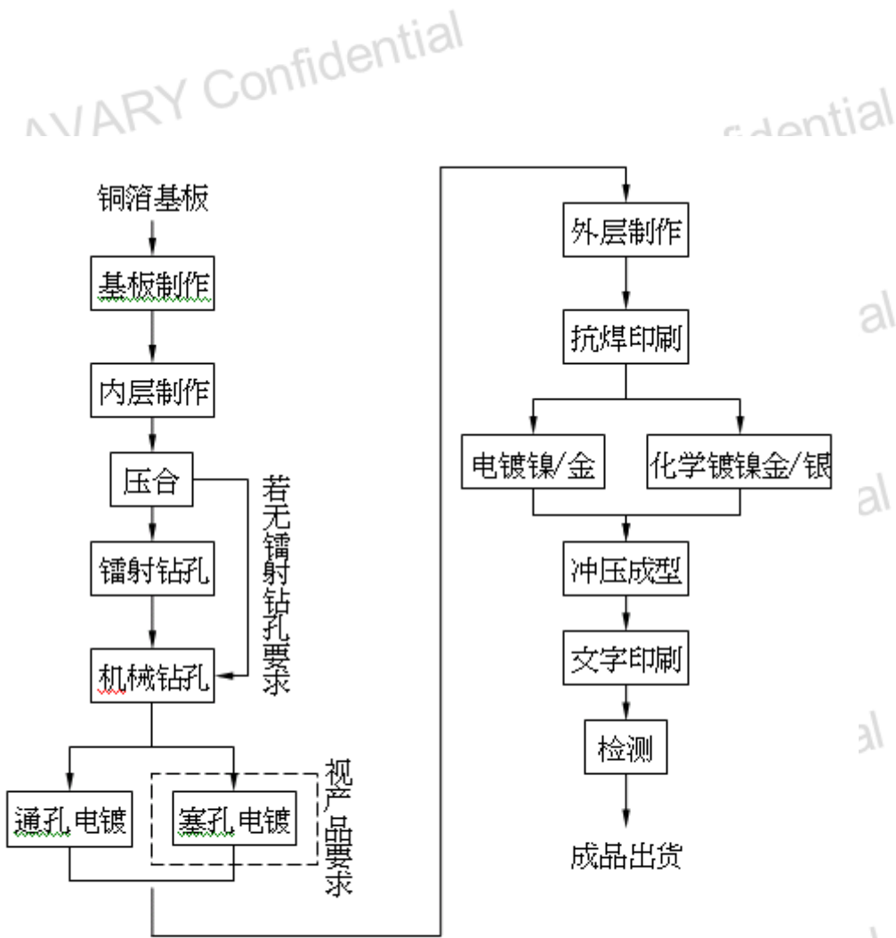
线路板总体工艺流程
